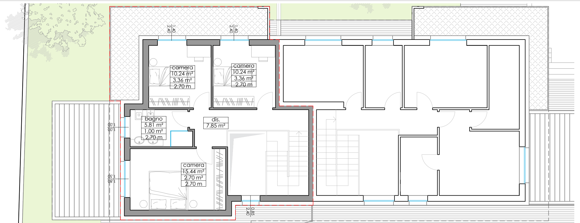
PIANO PRIMO SCALA 1:100
