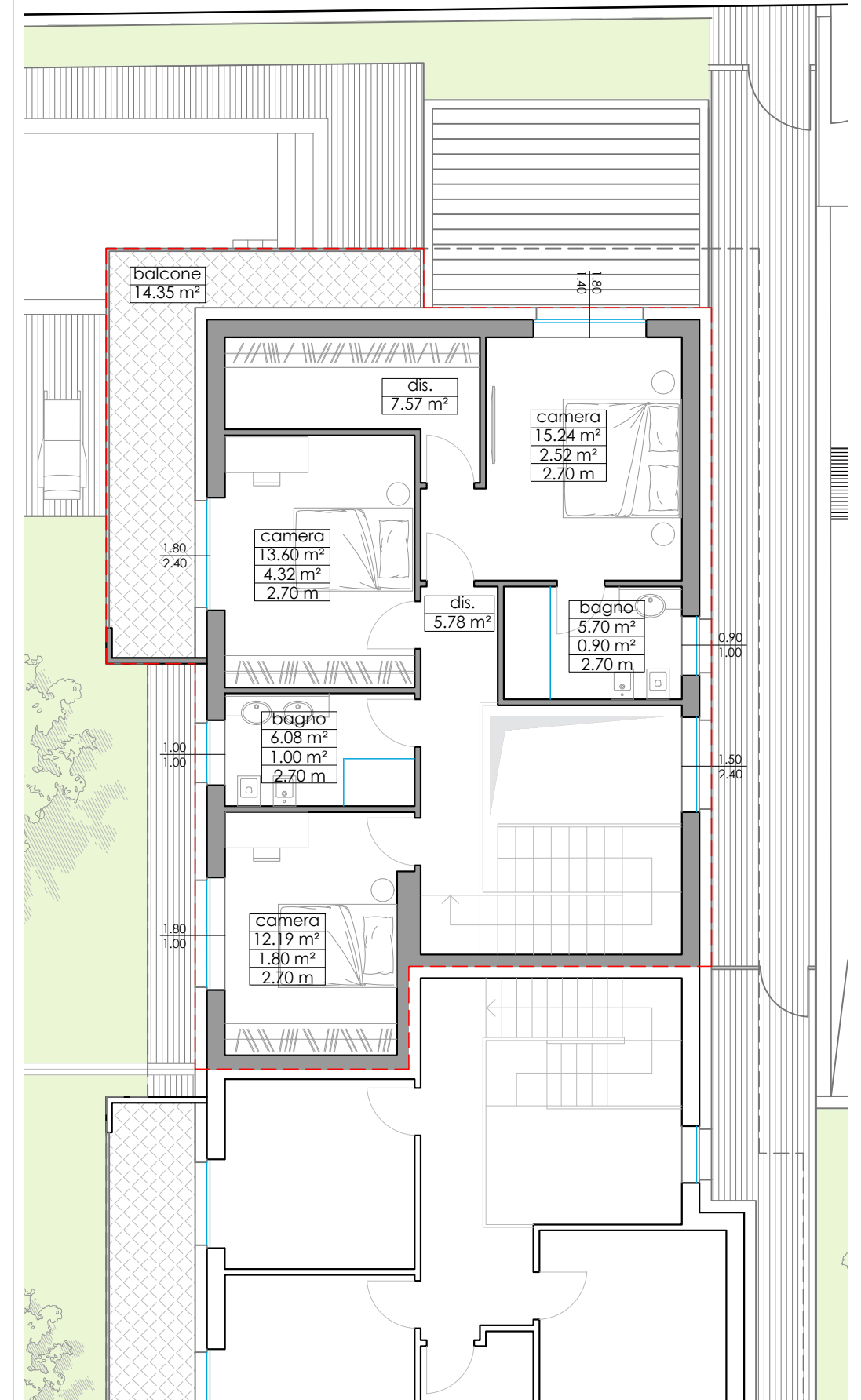
PIANO PIANO PRIMO SCALA 1:100
